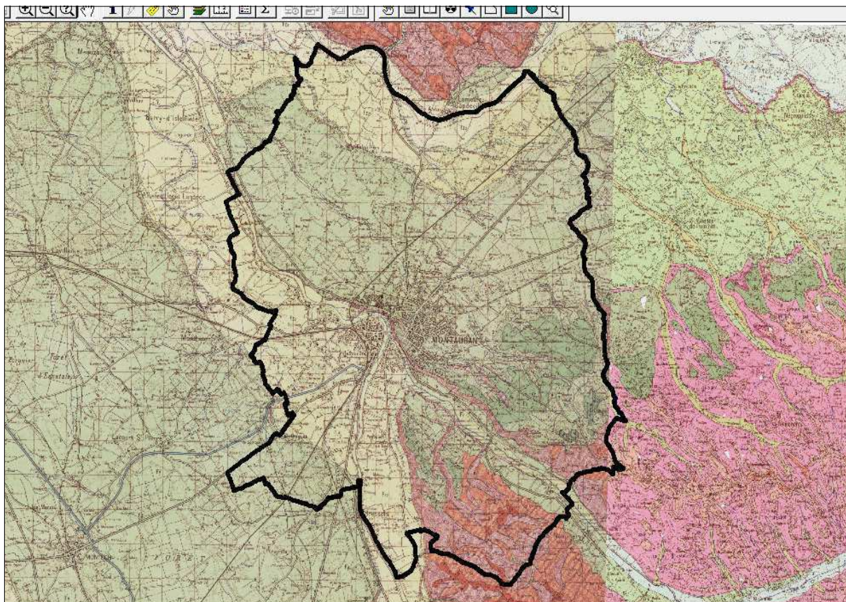
Figure 6 : Carte géologique de la commune de MONTAUBAN [Source : BRGM]
