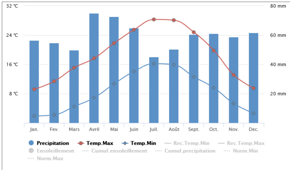
Figure 7 : Données climatiques de la station de MONTAUBAN [Source : www.meteofrance.com ]
